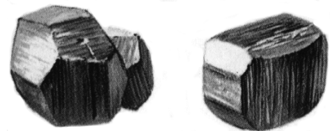
Pyriet kristallen
